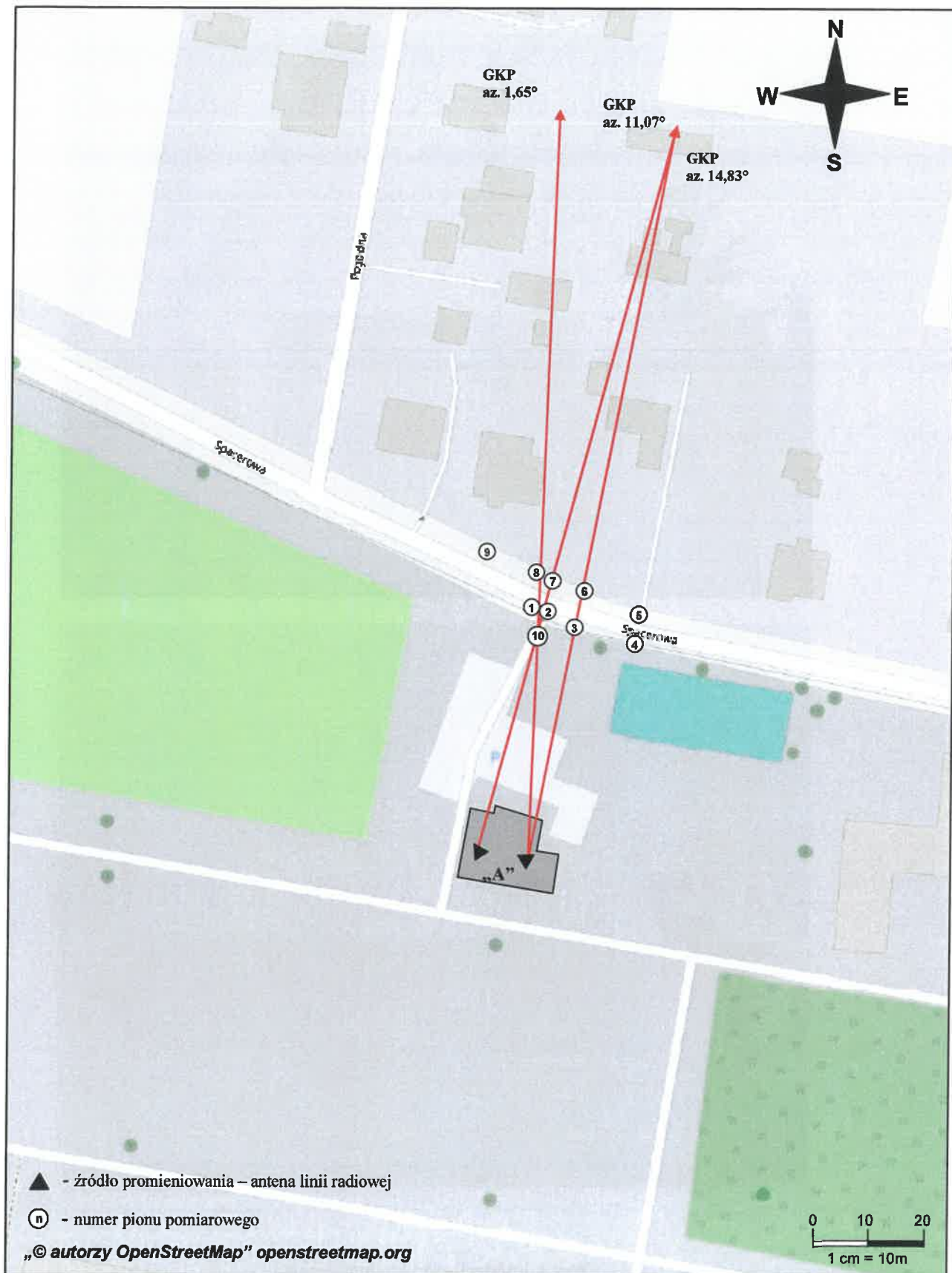
Rys. 1. Usytuowanie punktów i pionów pomiarowych w otoczeniu instalacji radiokomunikacyjnej Stacja Netia TERNB005-TERNM00003 Paprotnia, ul. Spacerowa 17
